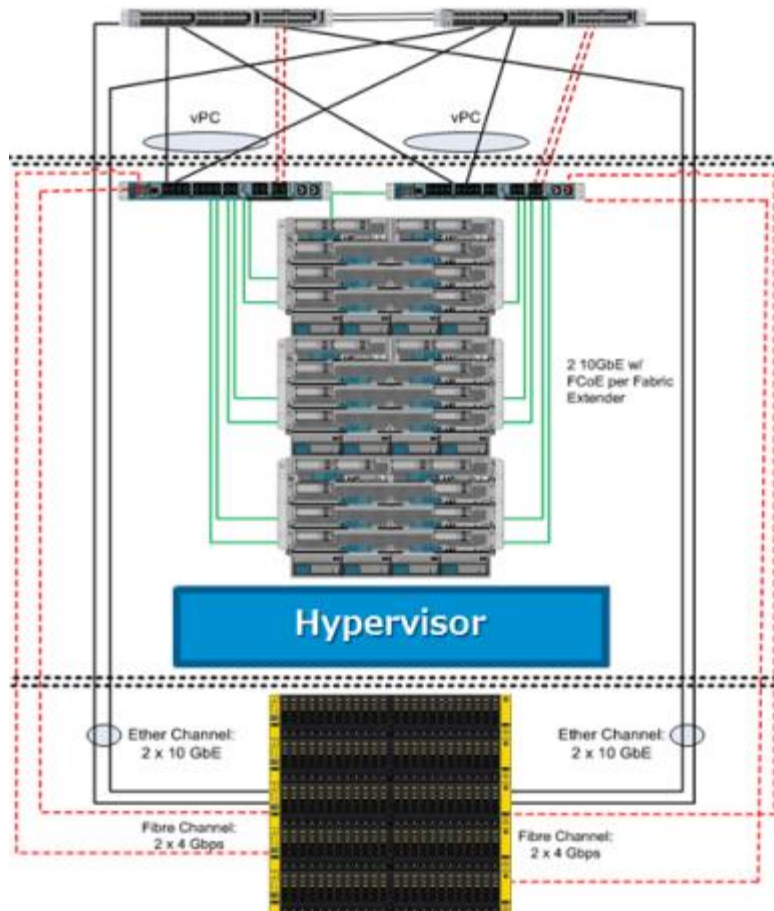
図6 サーバとストレージ
