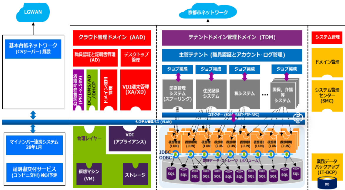
図7 基幹基盤の論理構成図
