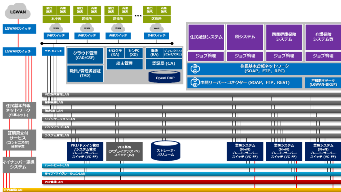
図9 ネットワーク構成概念図
