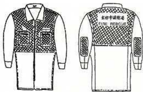
救助活動服上衣制式の図
