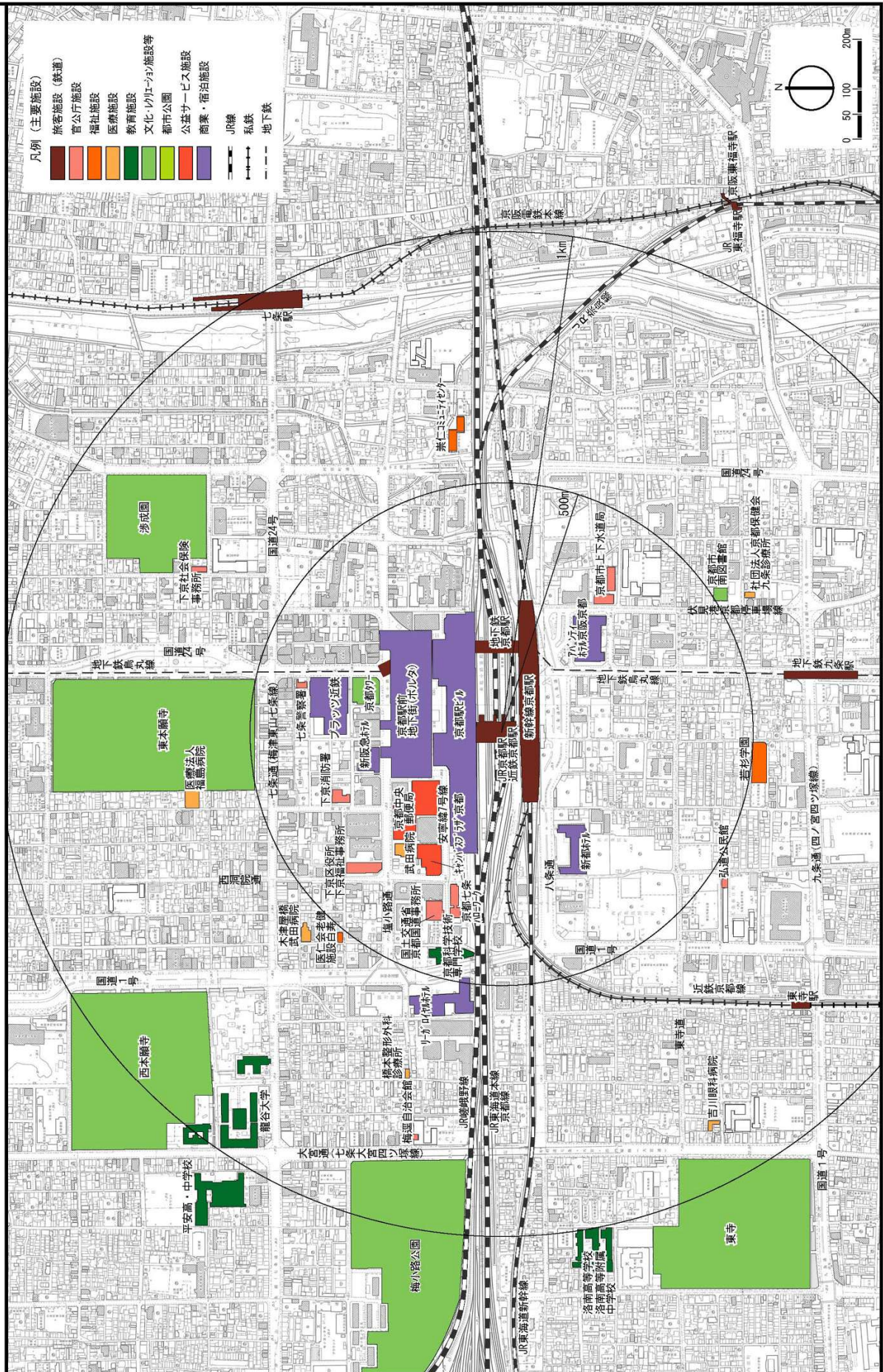
図-5 京都地区区内の施設の立地状況
